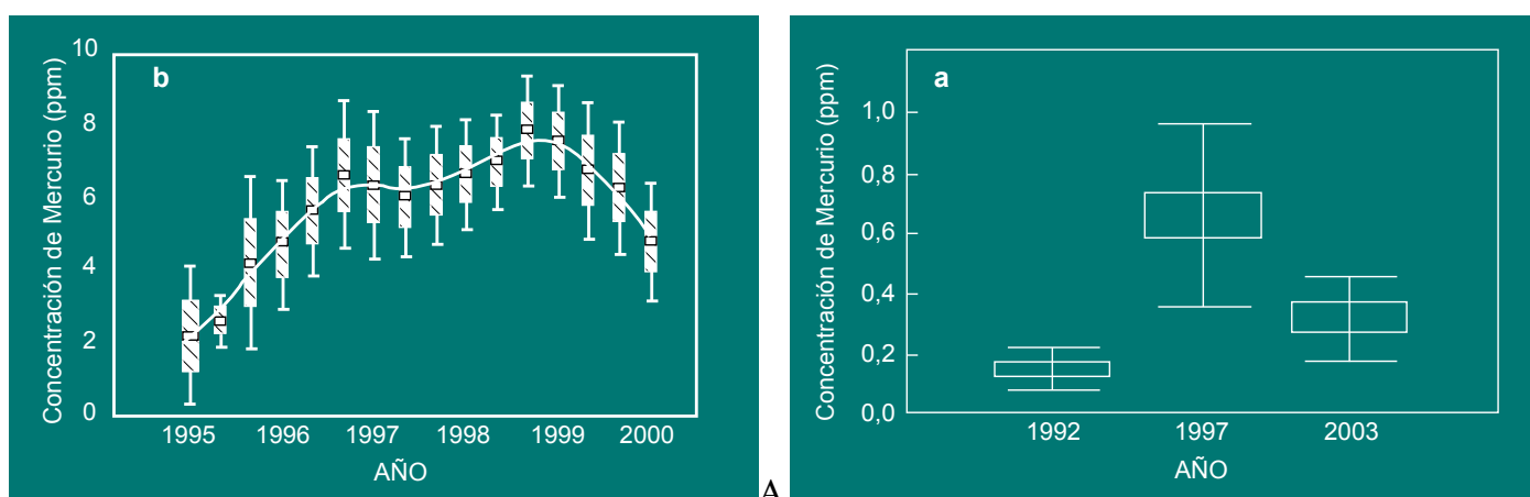
Figura 1.a) Variación histórica de los niveles promedio de mercurio en pez depredador ( Cichla spp) (Fuente: Forsberg, datos no publicados) y Figura 1.b) cabello humano en el reservorio Balbina (Wiesser et al. 2001).
